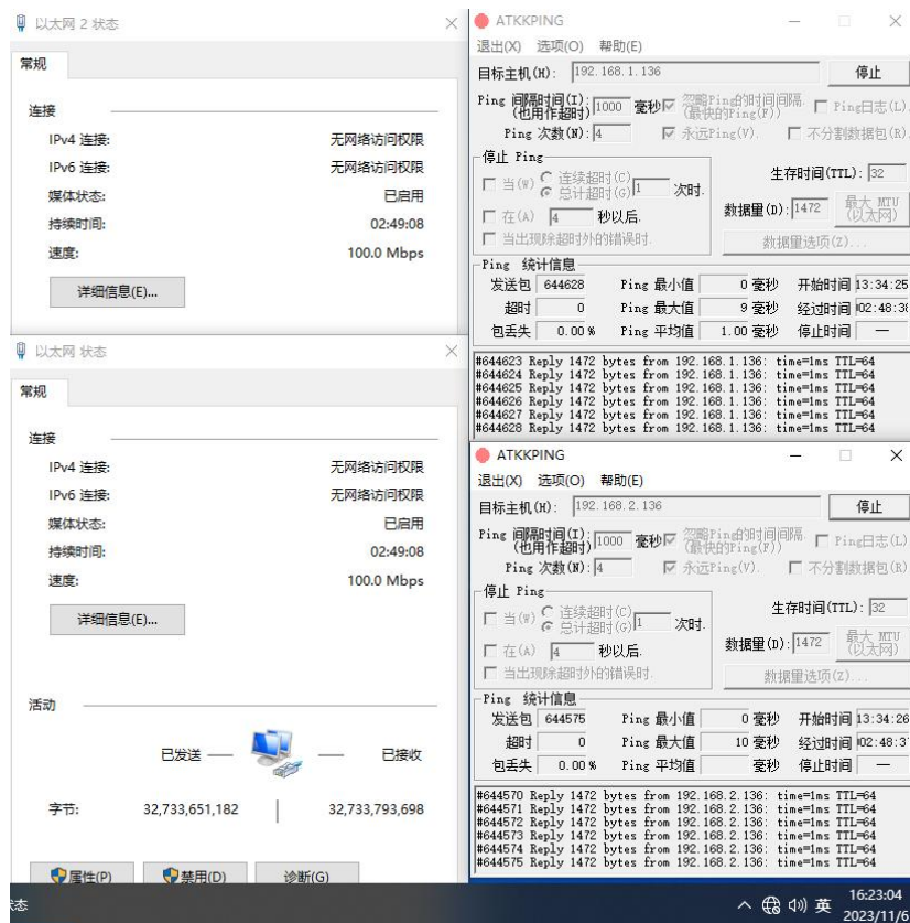
图 10 样机在高温试验时第一次启动运行检查功能正常
