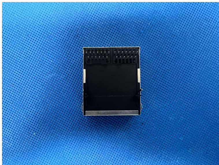
图 6 样机后视图
