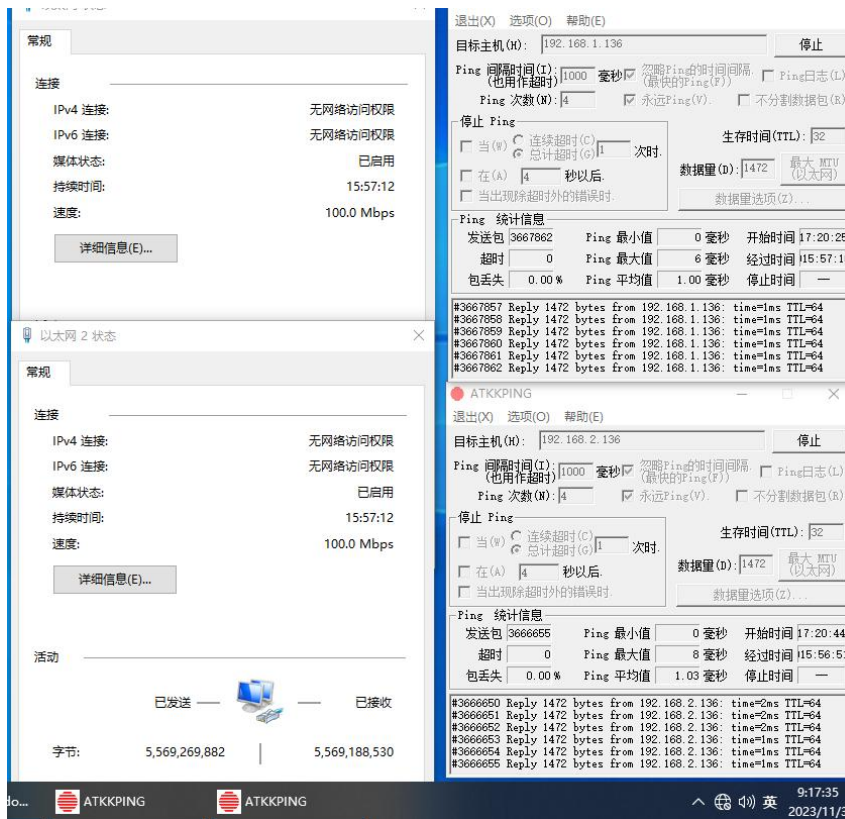
图 14 样机在湿热试验时第一次检查功能正常
