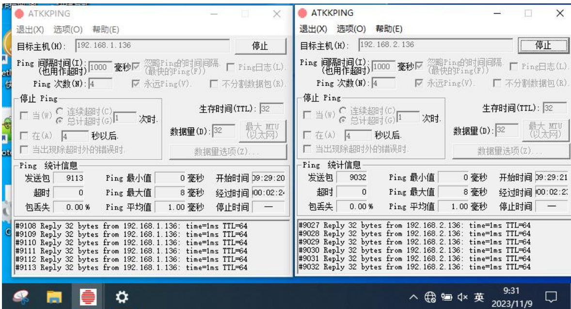
图 8 样机在低温试验时第二次启动运行检查功能正常
