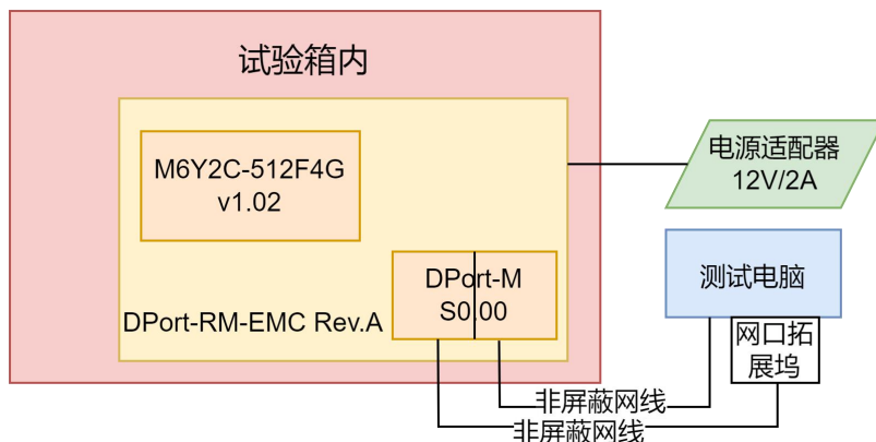
图 2 试验配置框图
