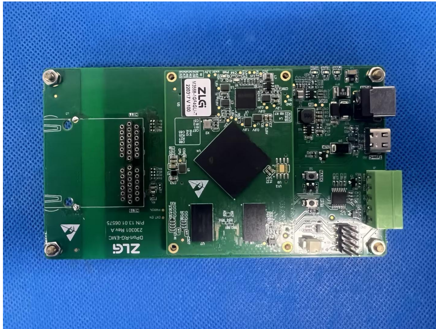
图 7 底板正视图
