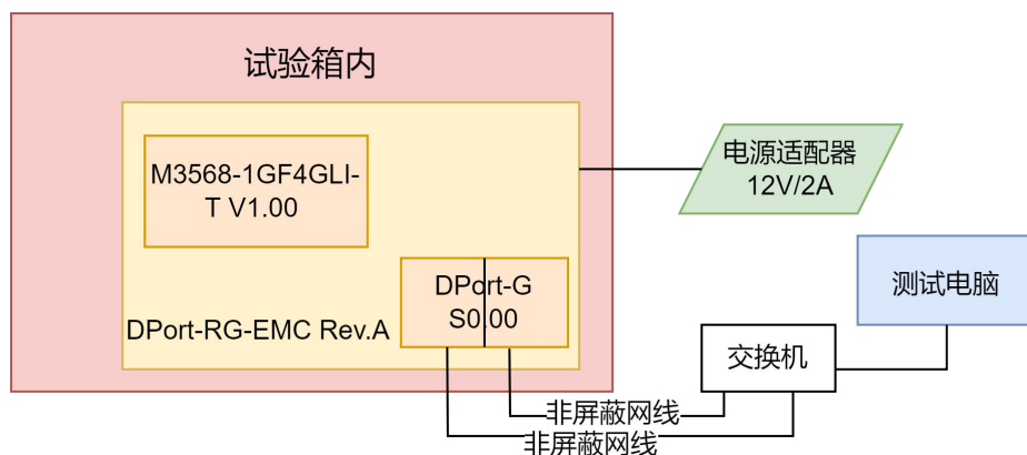
图 2 试验配置框图
