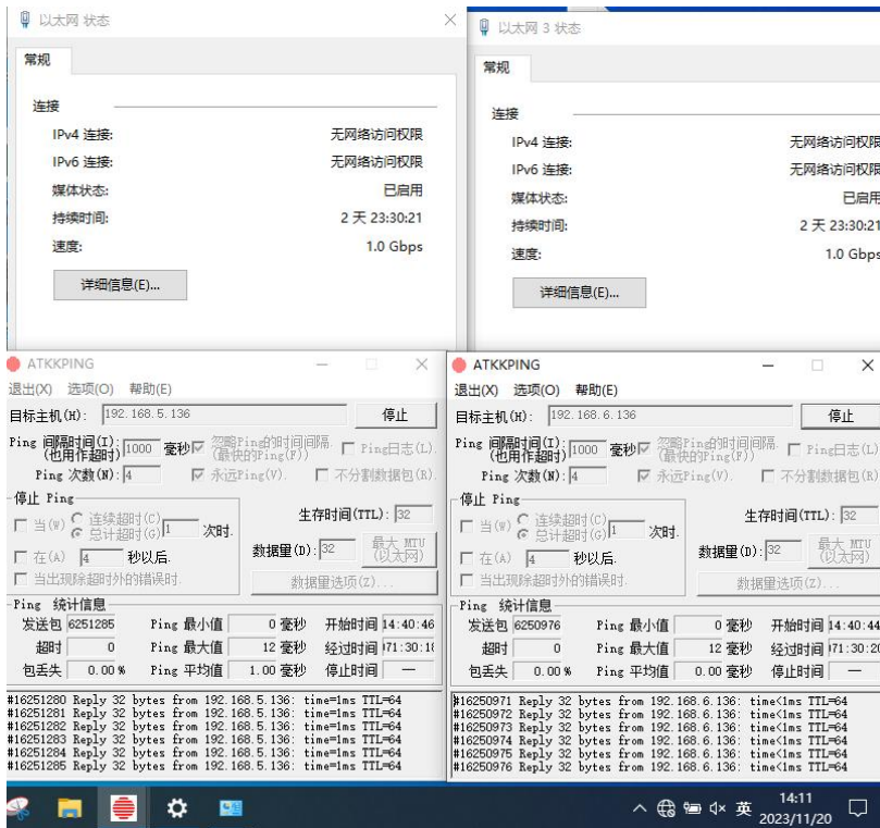
图 12 样机在高温试验时第一次启动运行检查功能正常
