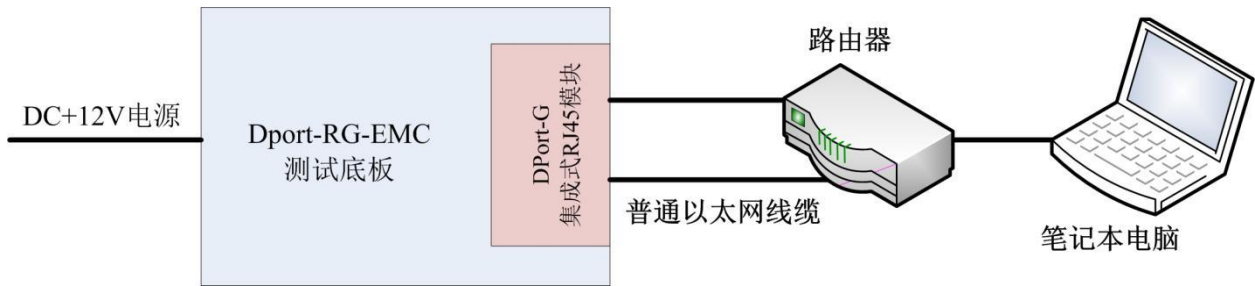
试验配置示意图
