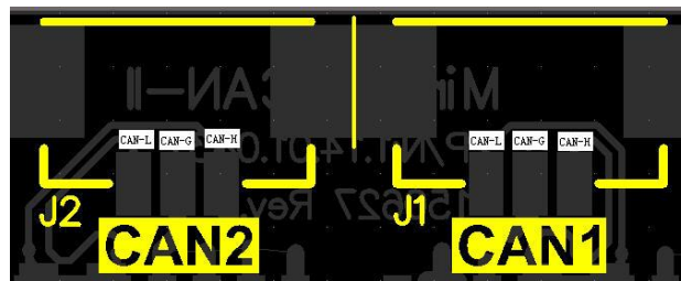
图 4.8 接口定义
