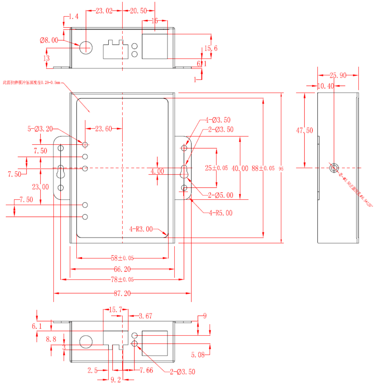
图 1.2 CANWiFi-200T 安装机械尺寸
