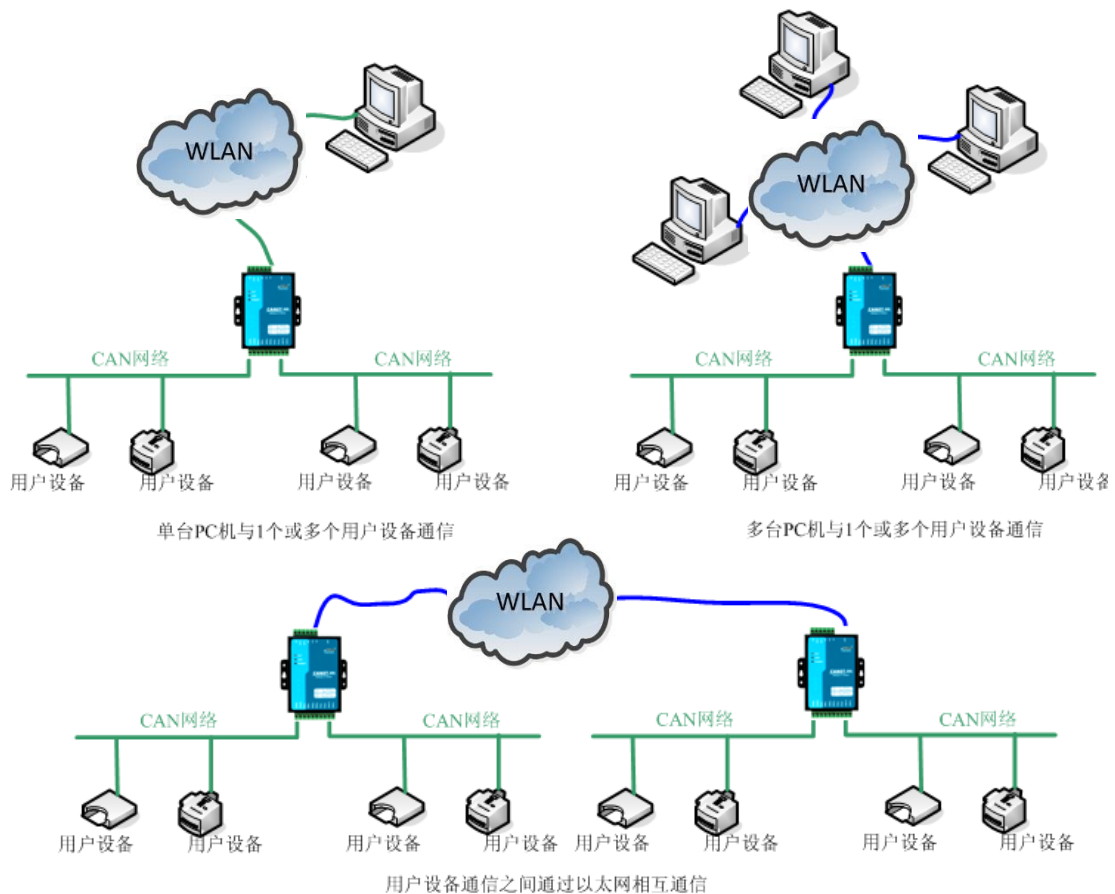
图 1.1 CANWiFi 典型应用图
