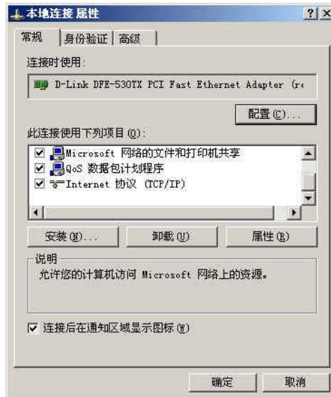
图 3.4 网络属性
