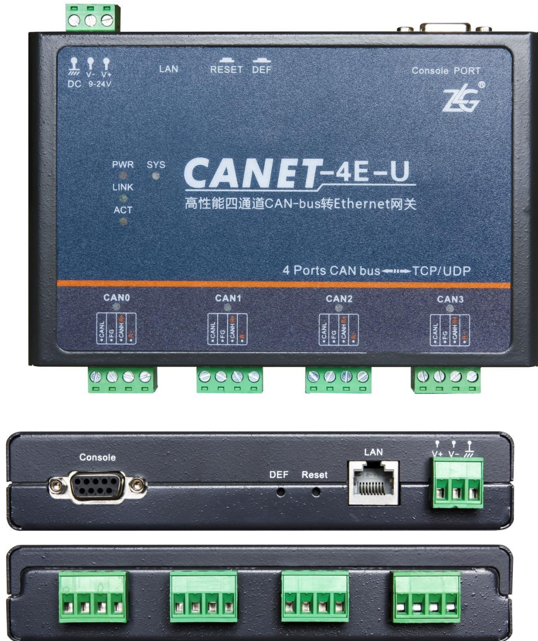
图 2.1 CANET-4E-U 外观图
