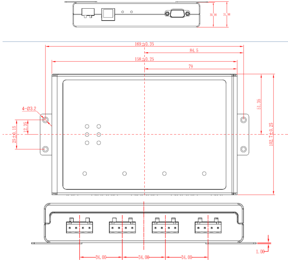
图 1.2 CANET-4E-U 安装机械尺寸
