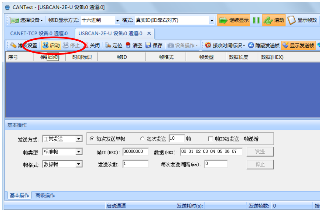
图 4.17 启动 USBCAN 卡
