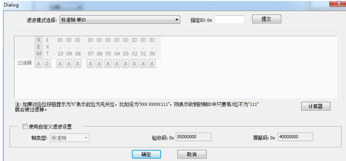
图 4.16 滤波计算器
