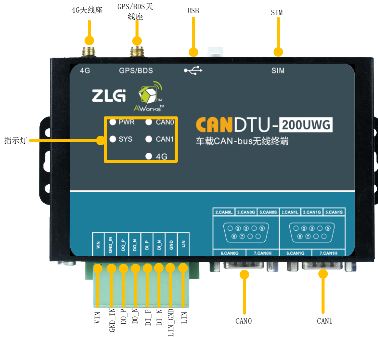
图 3.1 面板布局
