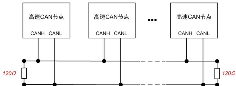
图 3.4 高速 CAN 典型网络连接示意图
