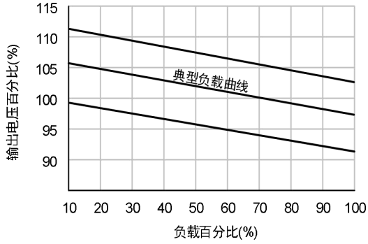
输出电压与负载关系曲线图 (标称输入电压)
